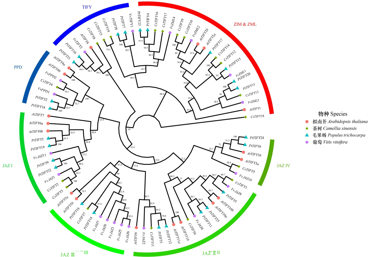
图 1 茶树、葡萄、毛果杨和拟南芥的 TIFY 基因家族系统发育树及其分类(Bootstrap 重复数为 1 000 次)
