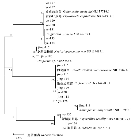
图 2 NJ 法构建的夹竹桃内生真菌 ITS 序列系统进化树图
