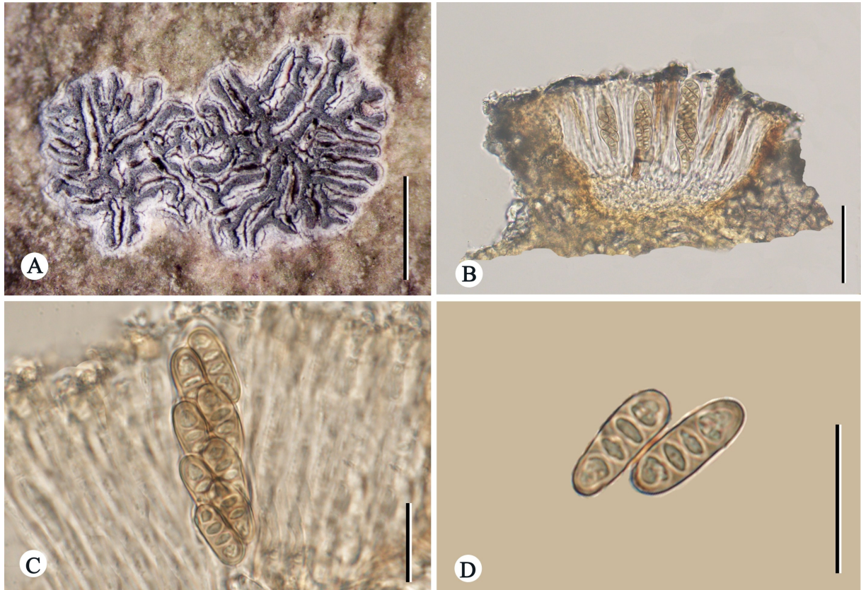
标尺: A=1 mm; B=50 \mu\text{m} ; C=20 \mu\text{m} ; D=20 \mu\text{m} 。 Bars: A=1 mm; B=50 \mu\text{m} ; C=20 \mu\text{m} ; D=20 \mu\text{m} 。
