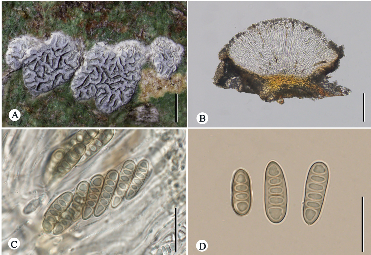
A. 地衣体和子囊器；B. 子囊盘横切面；C. 子囊；D. 子囊孢子。下同。标尺：A=1 mm；B=100 \mu\text{m} ；C=20 \mu\text{m} ；D=20 \mu\text{m} 。 A. Thallus with ascomata；B. A cross section of apothecium；C. Ascus；D. Ascospores. The same below. Bars：A=1 mm；B=100 \mu\text{m} ；C=20 \mu\text{m} ；D=20 \mu\text{m} .
