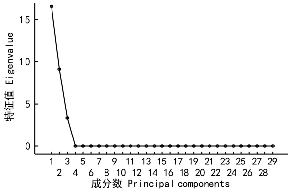
图 2 主成分的碎石图
