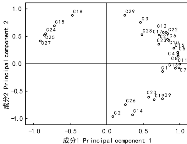
图 3 主成分载荷图
