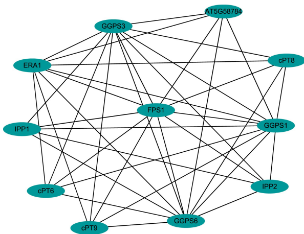
图 4 IcFPS1 蛋白质互作网络
