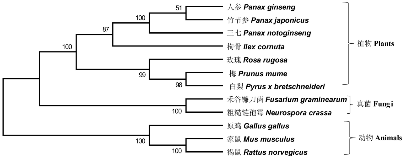
图 3 不同物种 FPS 基因的系统进化树
