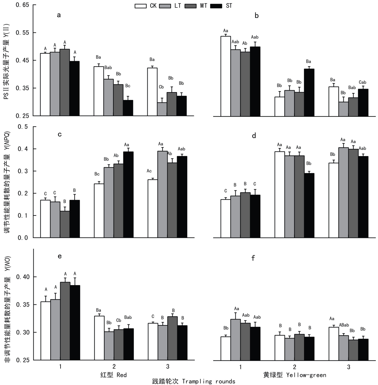
图 3 践踏对红型、黄绿型中位泥炭藓 Y(II) 、 Y(NPQ) 和 Y(NO) 的影响
