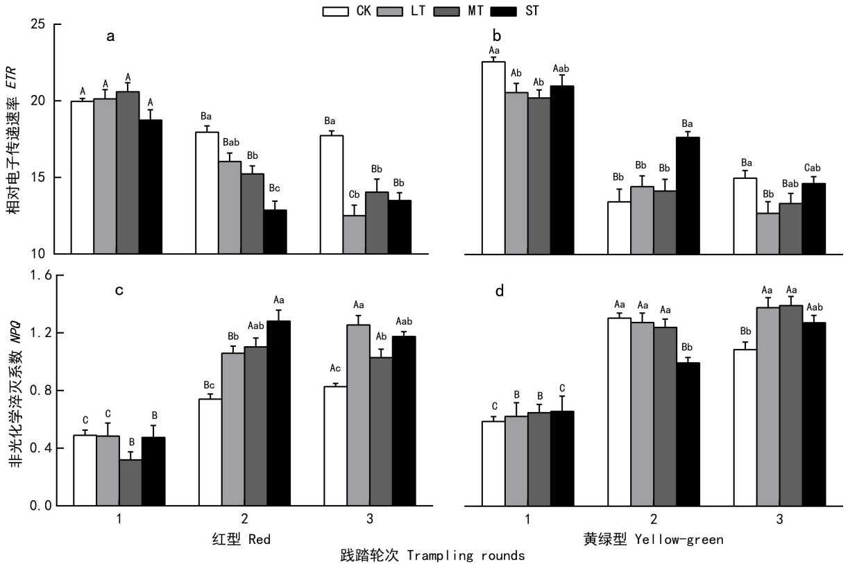
图 4 践踏胁迫对红型、黄绿型中位泥炭藓 ETR 和 NPQ 的影响
