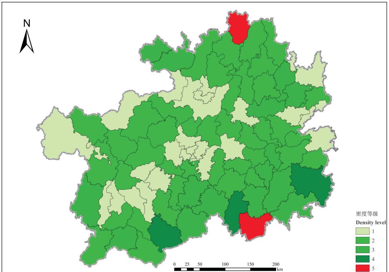
图 1 贵州省县域单元国家重点保护植物物种丰富度分布示意图
