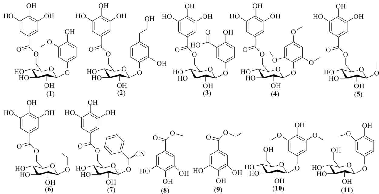
图 1 化合物 1-11 的结构
