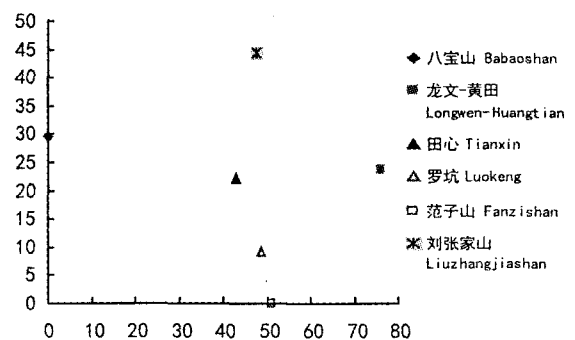
图 2 6 个森林群落的二维极点排序图
