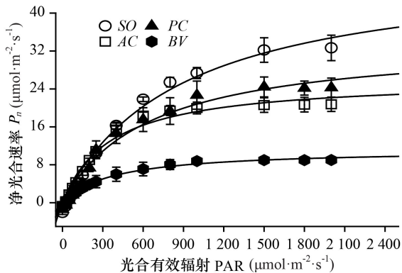
图 5 四种禾本科植物光响应曲线
