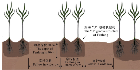
图 2 粉垄“145”模式甘蔗种植示意图
