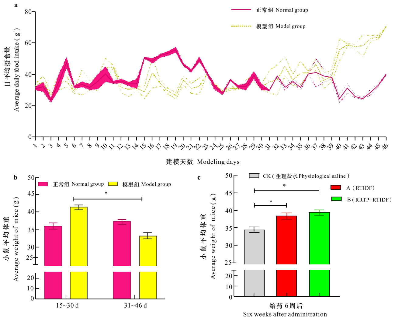
a. 建模过程小鼠日平均摄食量变化; b. 建模过程小鼠体重变化; c. 给药 6 周后小鼠体重变化。* 代表小组间的差异达到显著水平 ( P<0.05 )。
