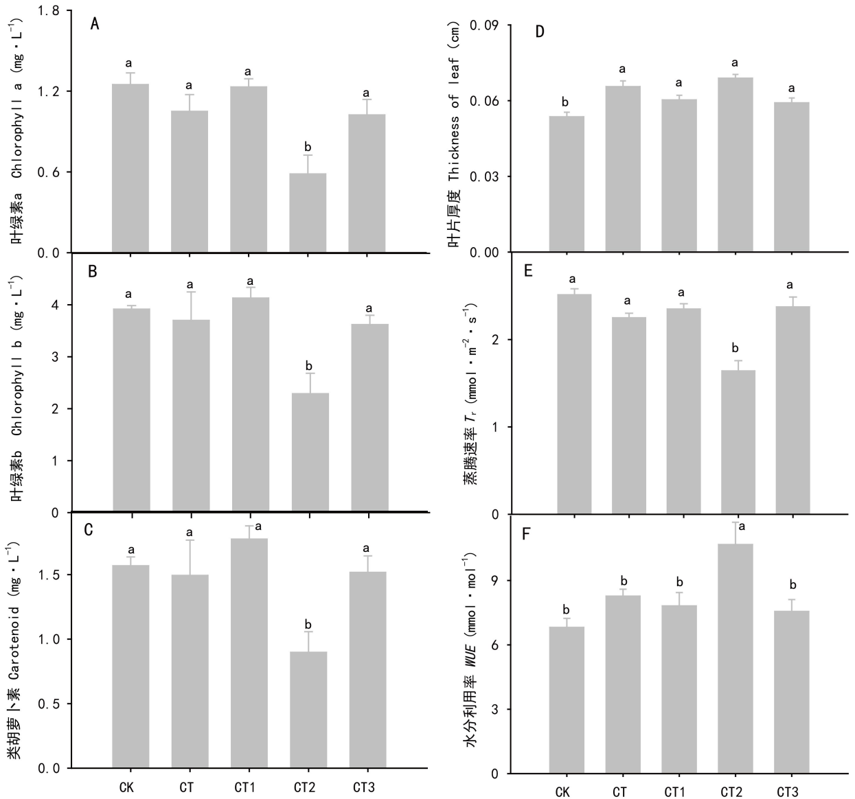
图3 绿甘蓝叶绿素 a 含量(A)、叶绿素 b 含量(B)和类胡萝卜素含量(C)、叶片厚度(D)、蒸腾速率(E)和水分利用效率(F)
