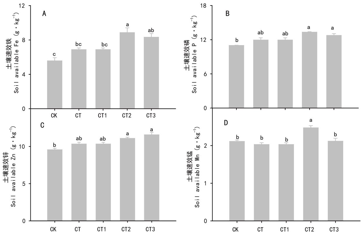
图 5 土壤速效铁(A)、速效磷(B)、速效锌(C)和速效锰(D)含量 Fig. 5 Contents of soil available iron (A), available phosphorus (B), available zink (C) and available manganese (D)
