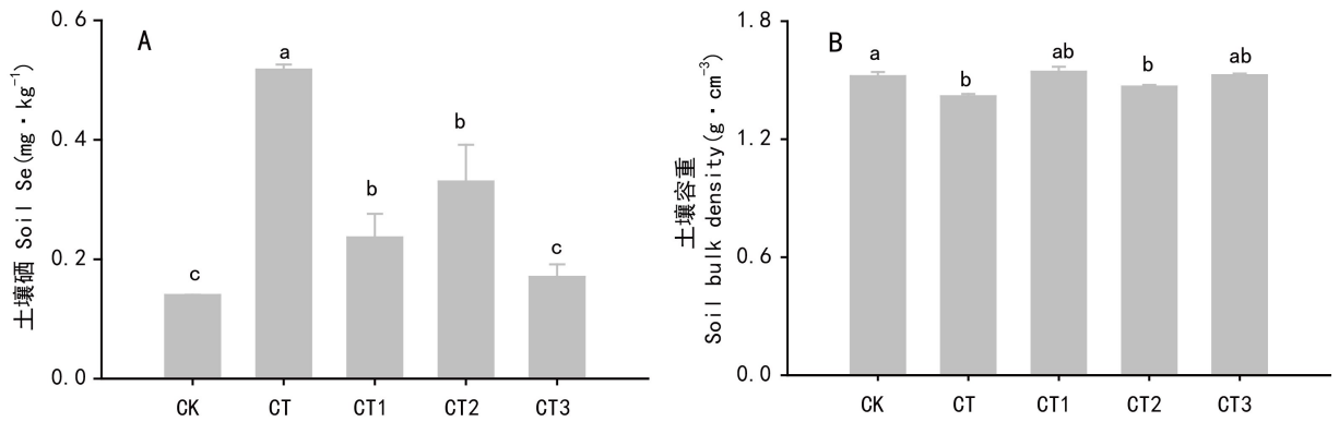
图 4 土壤硒含量(A)和土壤容重(B) Fig. 4 Soil Se content (A) and bulk density (B)
