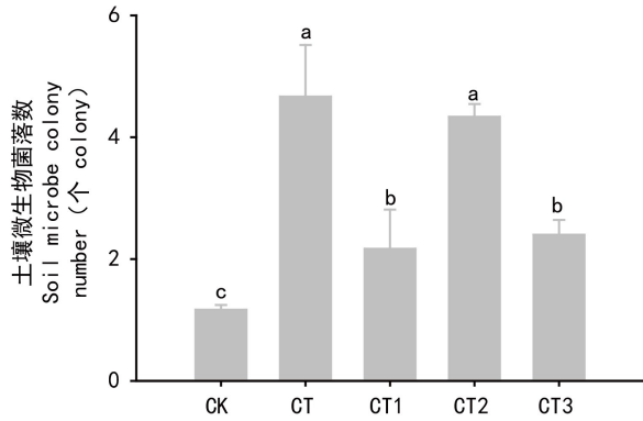
图 6 土壤微生物菌落数
