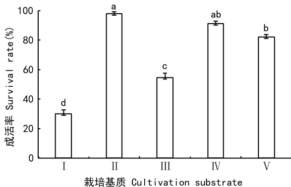
图 2 不同栽培基质对西藏虎头兰试管苗移栽成活率的影响
