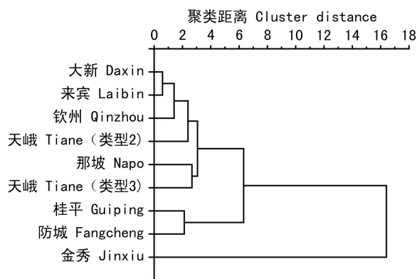
图 5 两面针样品聚类分析结果
