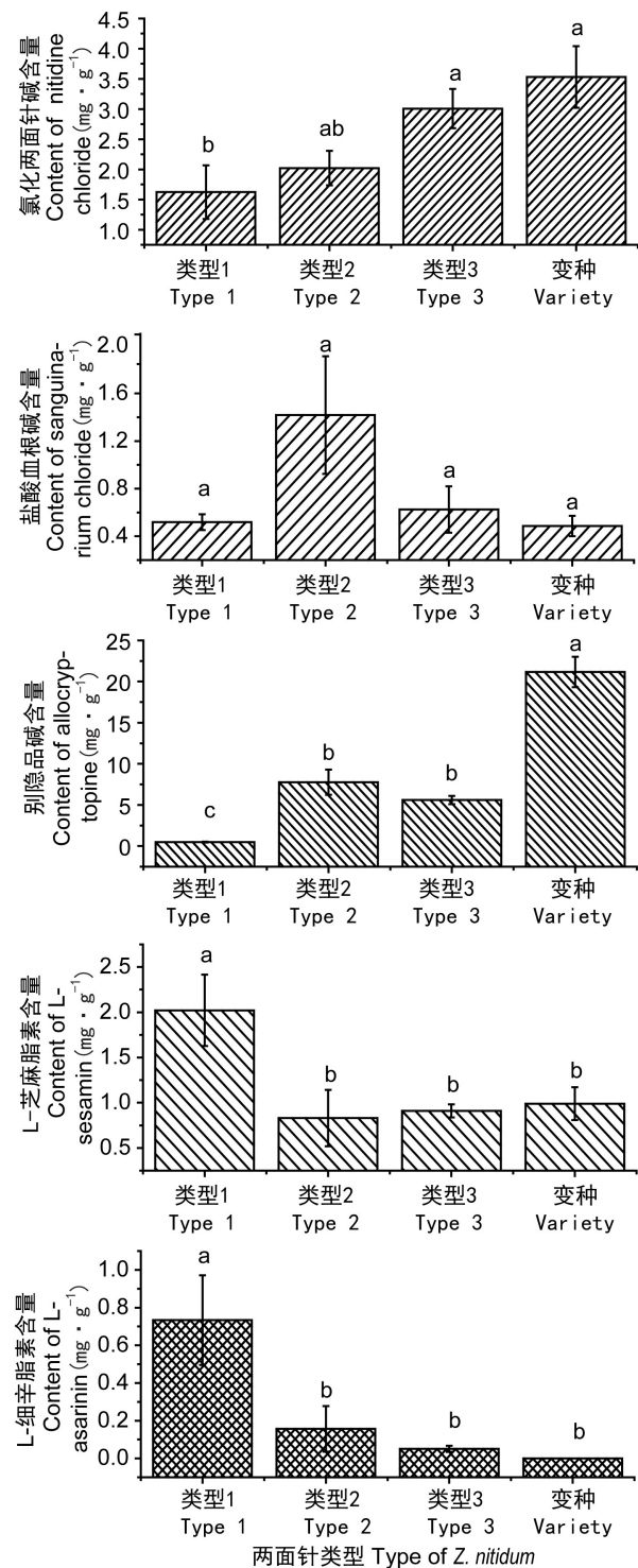
图4 不同产地及不同类型两面针含量测定结果及差异性分析
