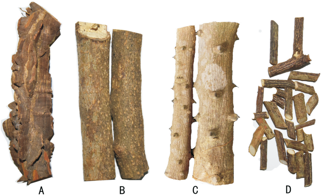
注: A. 两面针类型 1; B. 两面针类型 2; C. 两面针类型 3; D. 毛叶两面针。
