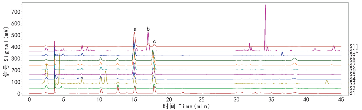
注: a. 氯化两面针碱; b. 毛两面针素; c. 白屈菜红碱与乙氧基白屈菜红碱。
