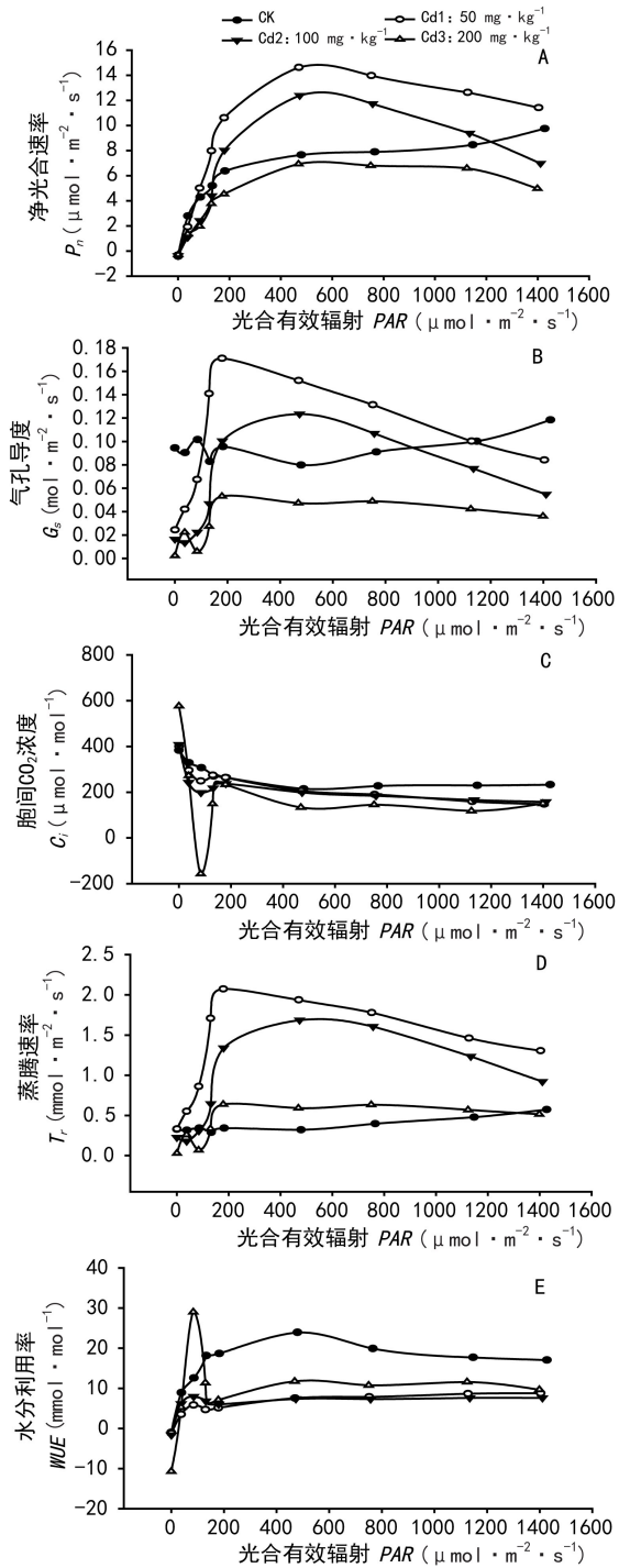
图 2 不同浓度 Cd 处理对芦竹光合作用的影响
