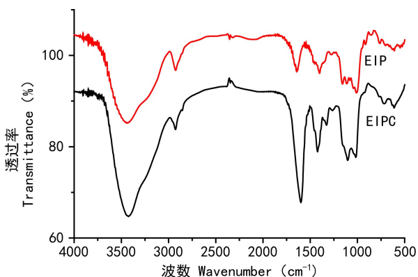
图 1 EIP 和 EIPC 红外光谱
