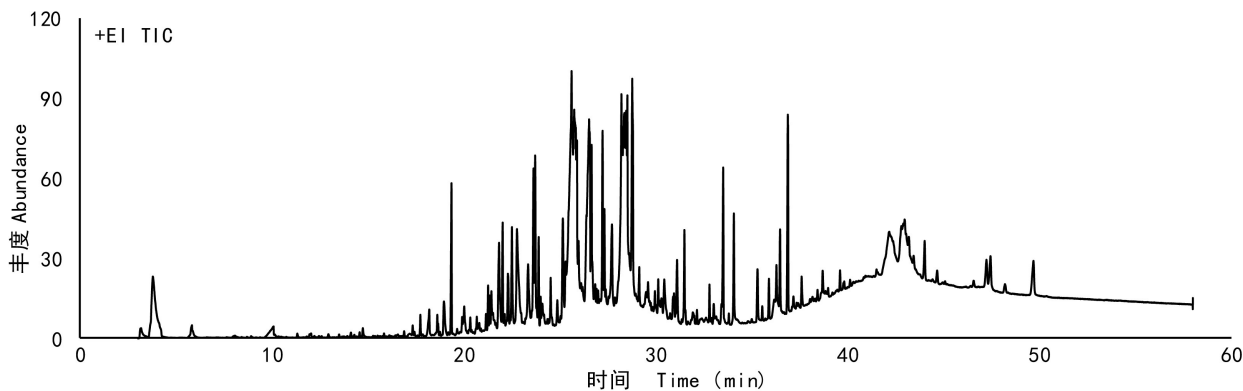
图 4 山芝麻根石油醚相萃取物的总离子流色谱图
