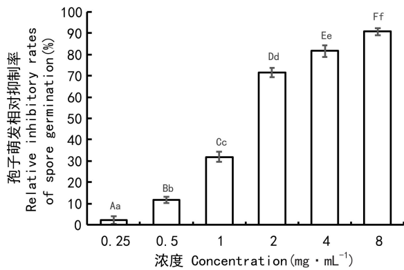
图 2 山芝麻根乙酸乙酯相萃取物对香蕉炭疽病菌分生孢子萌发相对抑制率
