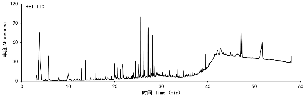
图 5 山芝麻根乙酸乙酯相萃取物的总离子流色谱图
