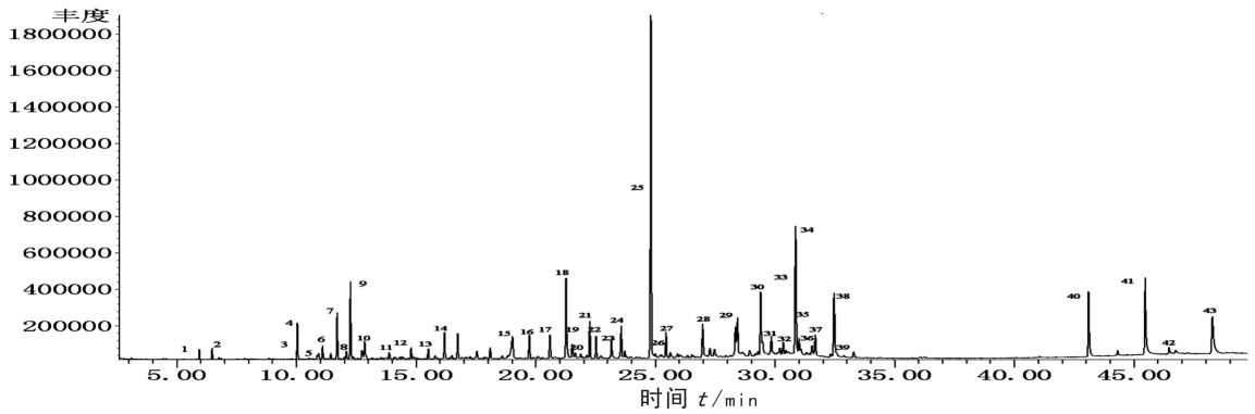
图 2 雪菊挥发油总离子色谱图
