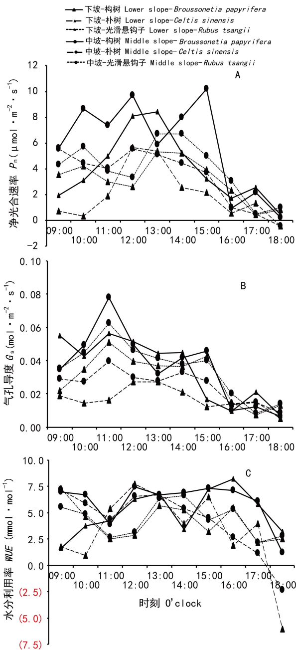
图 1 中坡位与下坡位三种植物的光合特性日变化 A. 净光合速率; B. 气孔导度; C. 水分利用效率。
