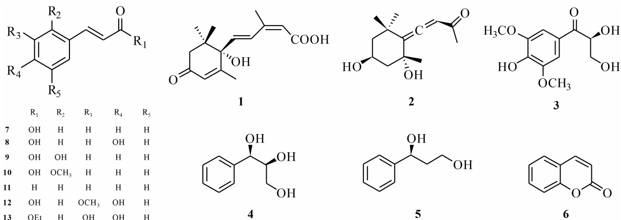
图1 化合物1-13结构 Fig. 1 Structures of compounds 1-13
