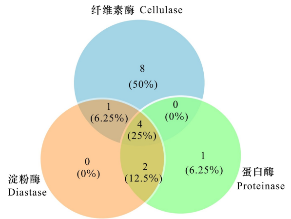
图 5 酶活性结果分析维恩图
