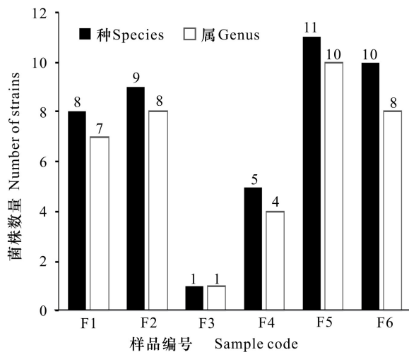
图 2 不同植物分离得到的可培养细菌分布情况
