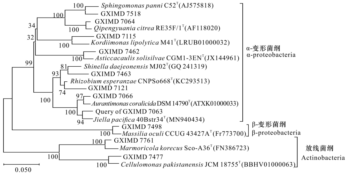
图 1 潜在新菌的 16S rRNA 基因序列 N-J 系统发育树
