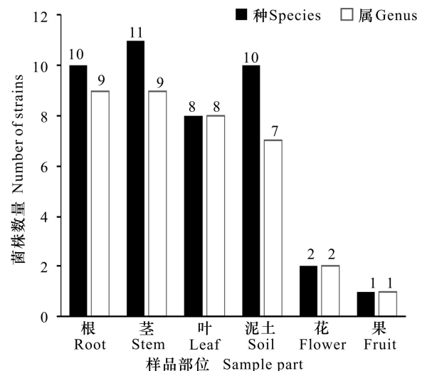
图 3 不同部位分离得到的可培养细菌分布情况
