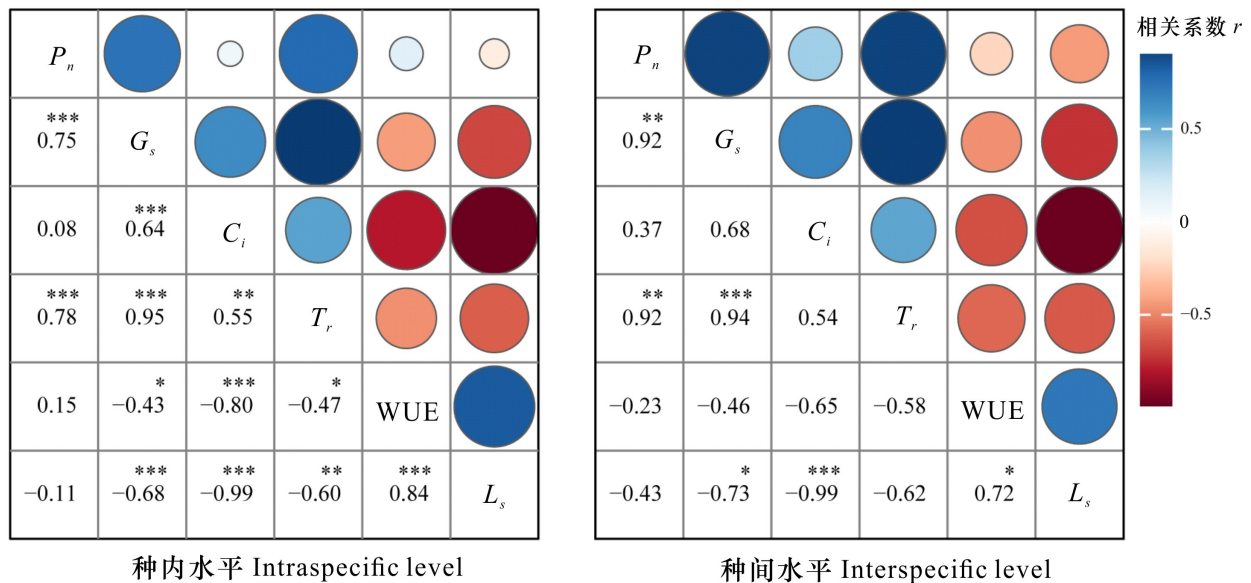
图 1 叶片光合特征参数在种内和种间水平上的 Pearson 相关系数
