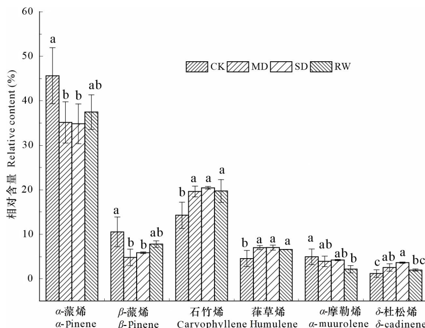
图3 干旱胁迫对抗旱型家系主要针叶挥发物的影响
