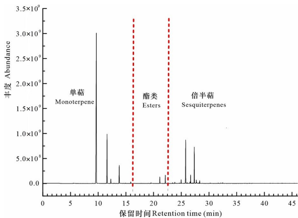
图 1 针叶挥发物 SPME-GC-MS 离子流图谱 Fig. 1 SPME-GC-MS ion chromatogram of needle volatiles
